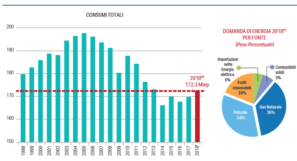
ITALIA Domanda di energia totale e per fonte (Milioni di tep)
