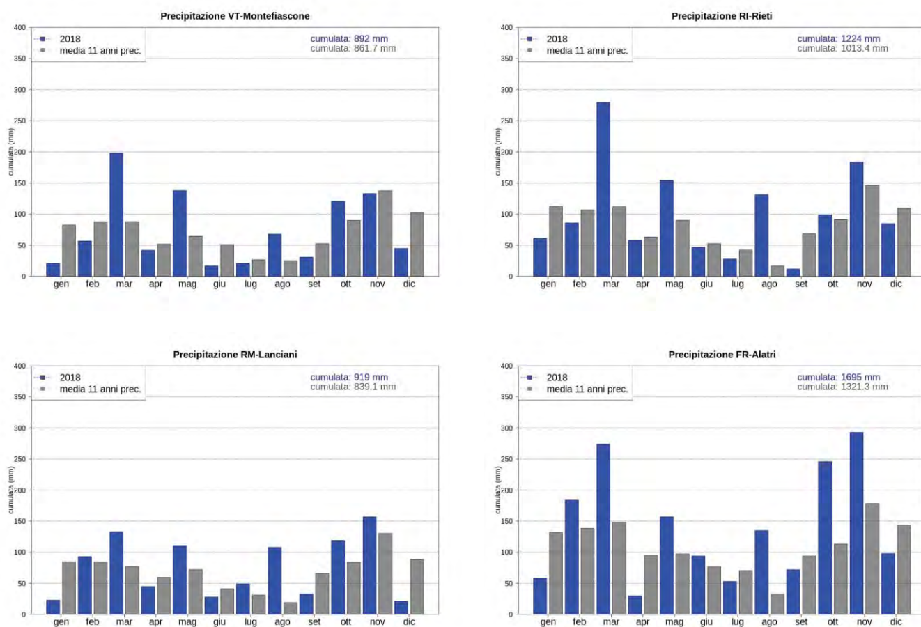
Figura 3-68 Istogramma mensile della precipitazione cumulata
