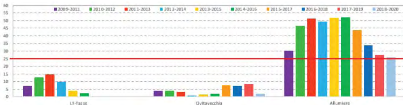
Figura 3-54 Superi media 8 ore dei 120 µg/m 3 zona Litoranea 2009-2020.
