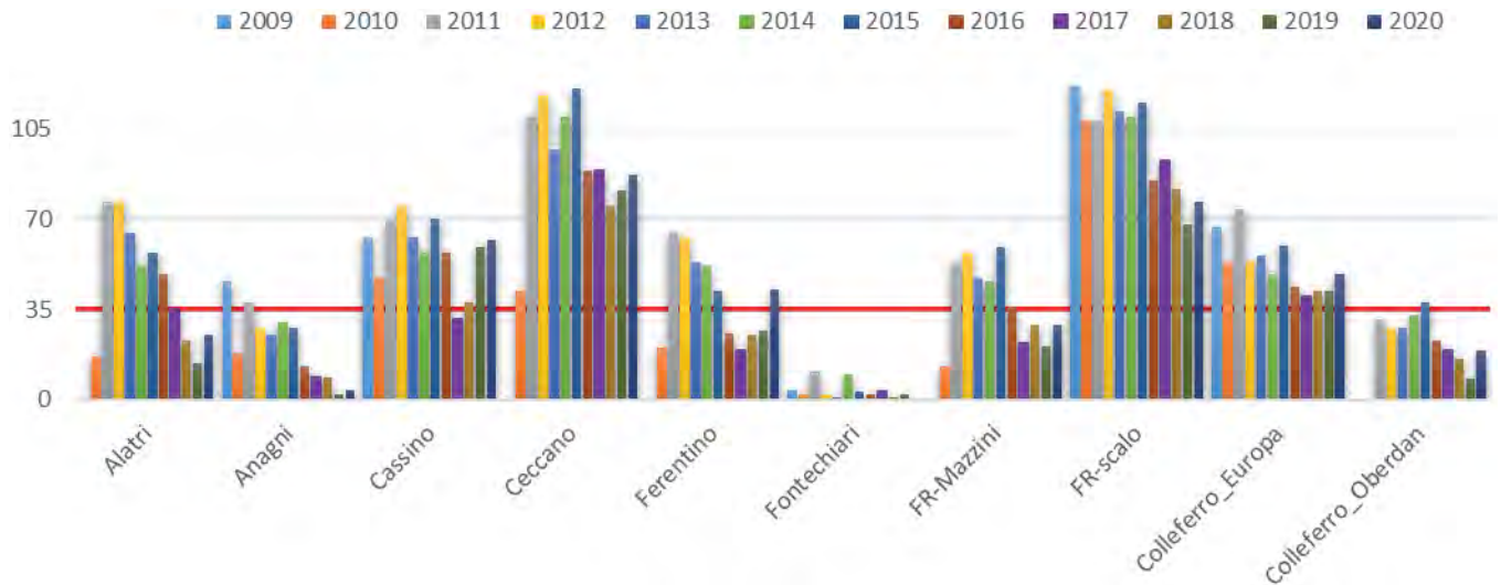
Figura 3-36 Superamenti valori limite giornaliero PM10 Zona Valle del Sacco 2009-2020.
