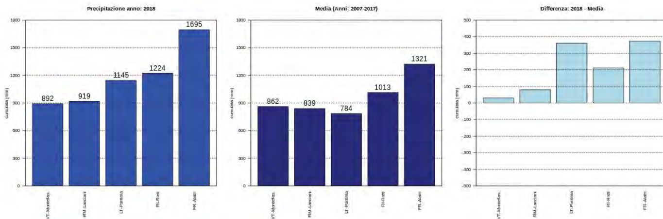
Figura 3-67 Istogrammi precipitazione
